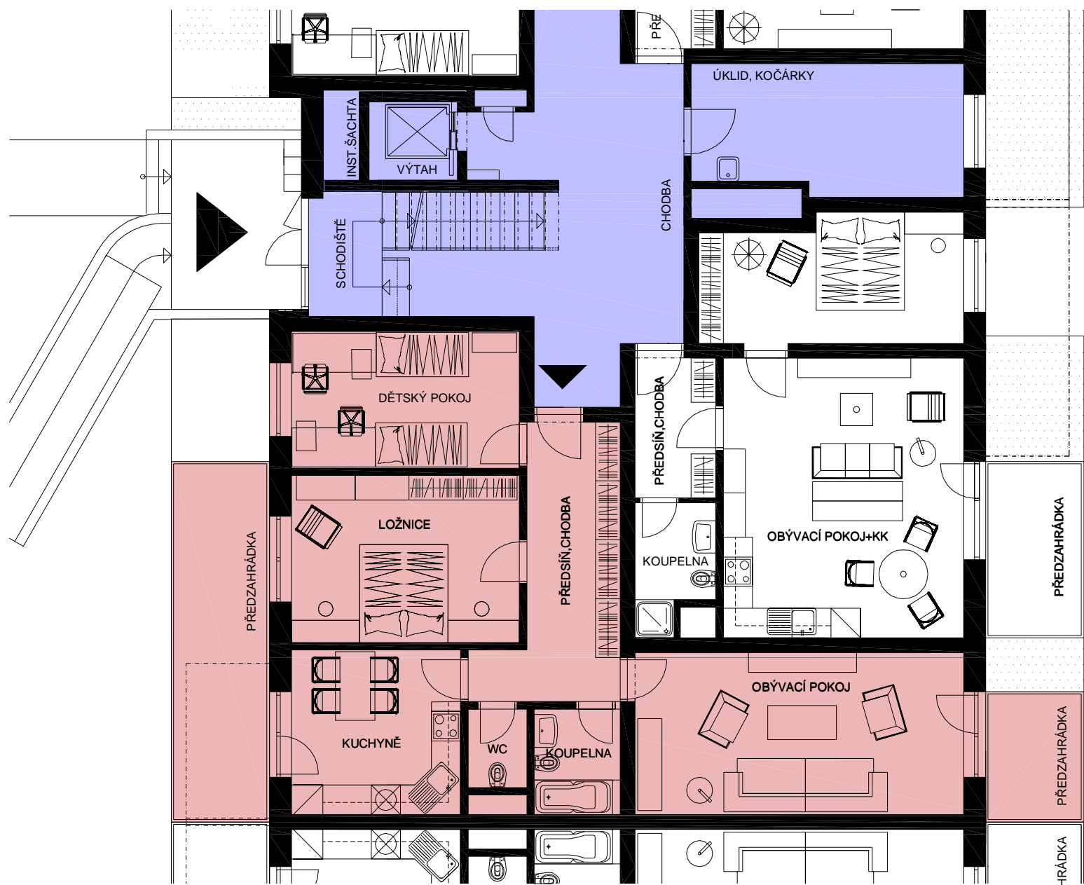
BYT 3+1 M2
